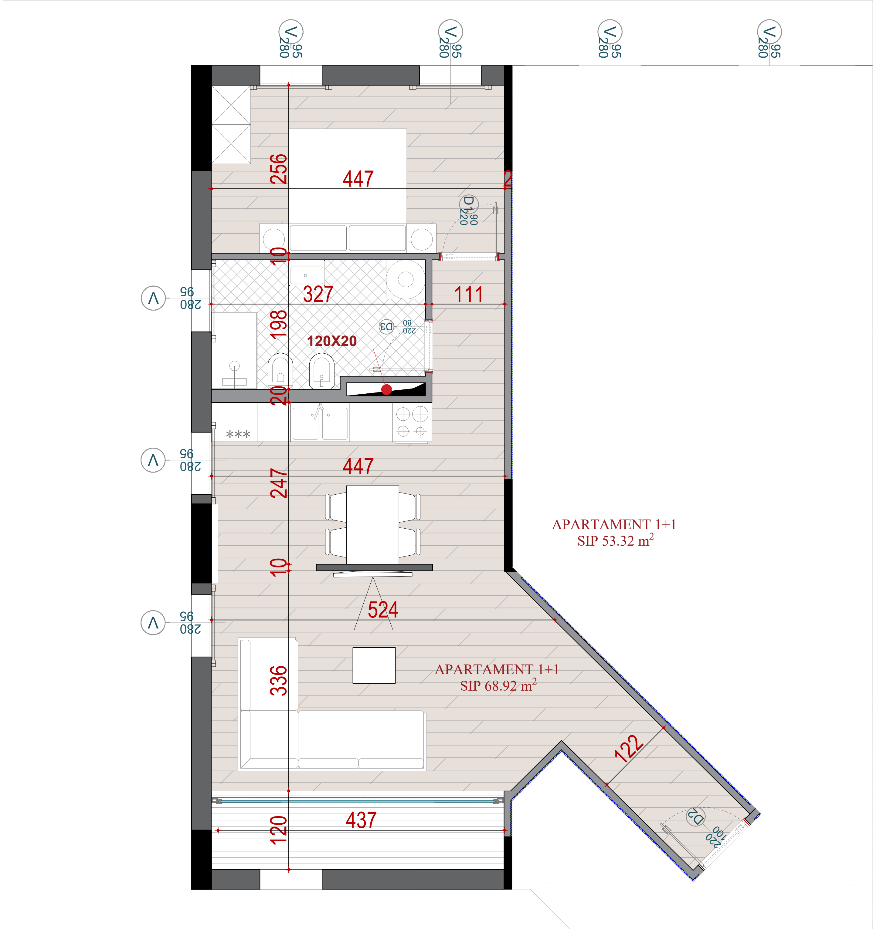
PLANIMETRIA E APARTAMENTIT NR. 44
