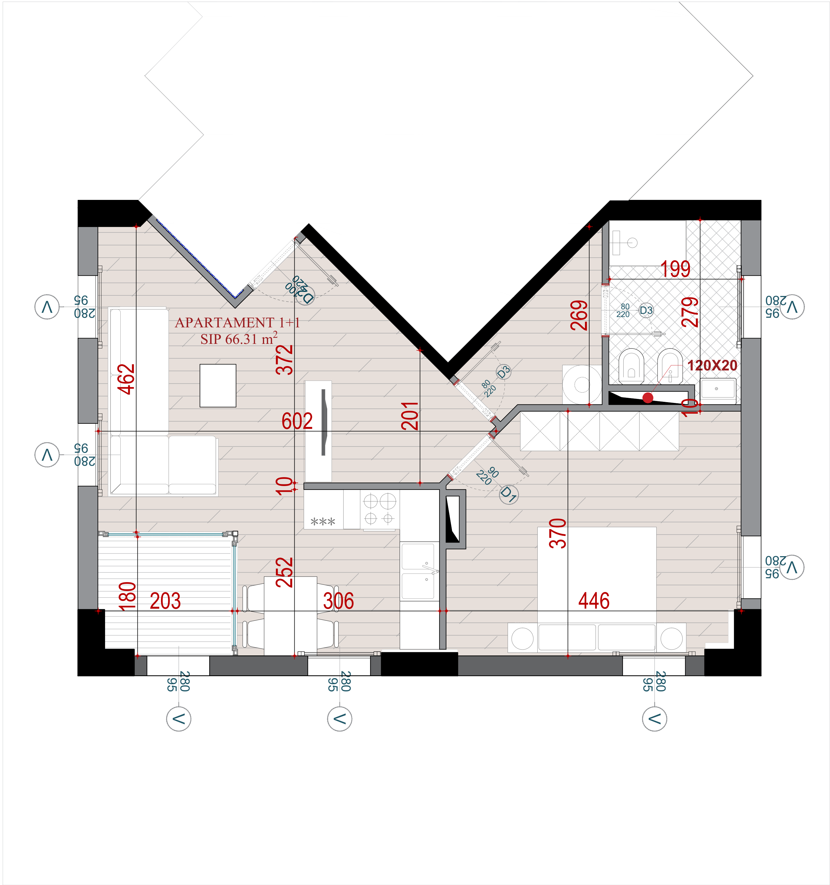
PLANIMETRIA E APARTAMENTIT NR. 43
