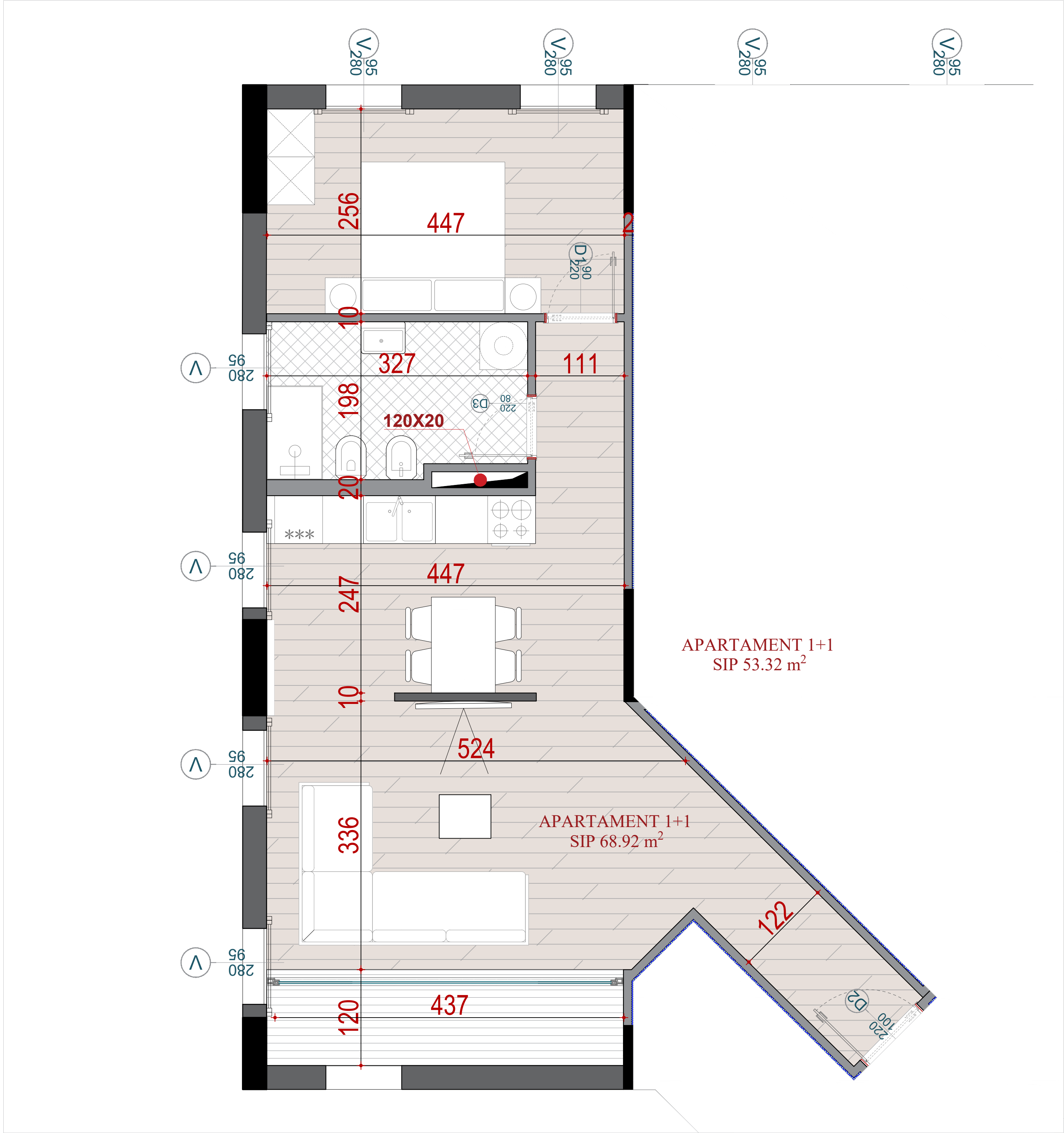
PLANIMETRIA E APARTAMENTIT NR. 40
