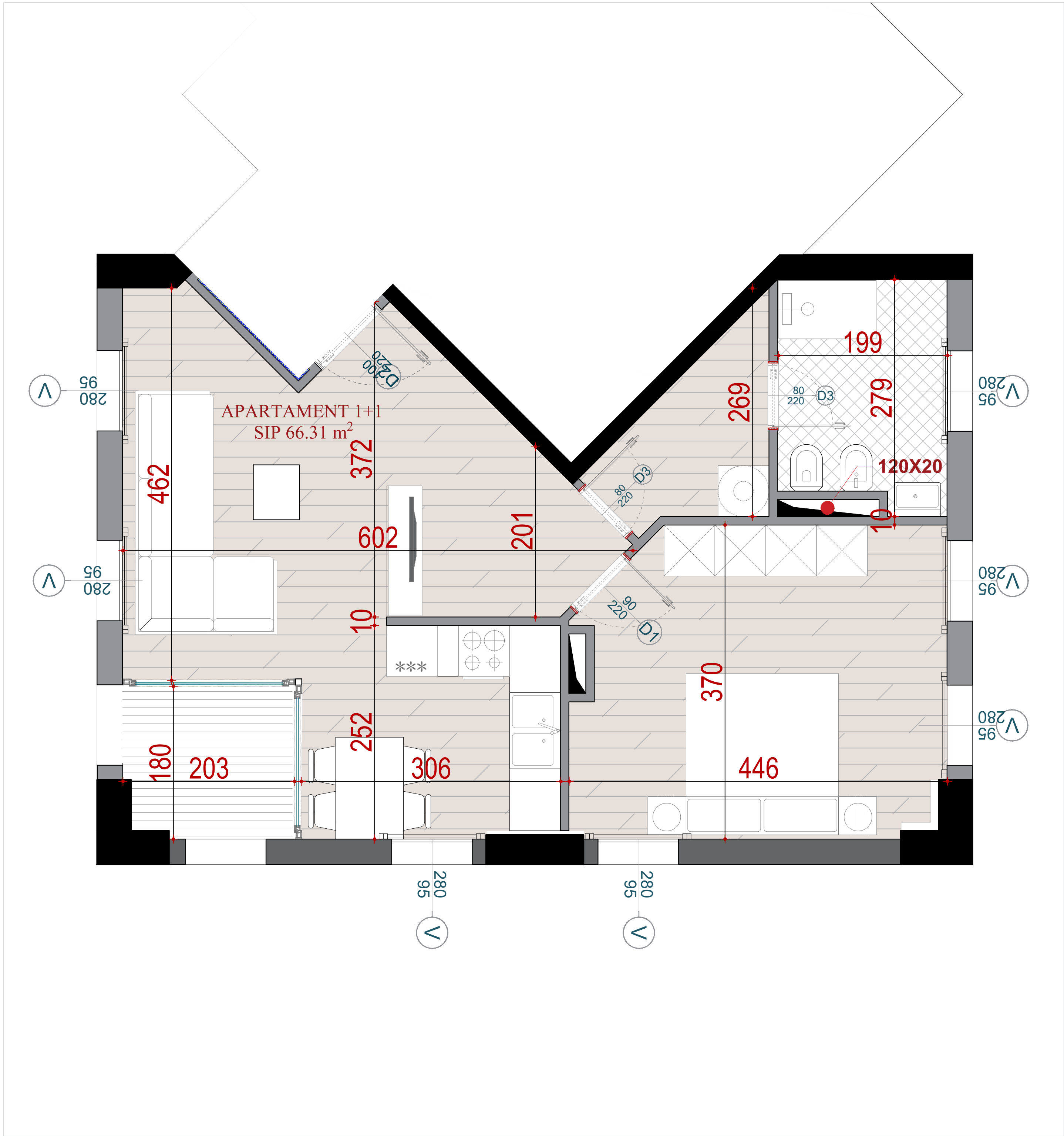
PLANIMETRIA E APARTAMENTIT NR. 39
