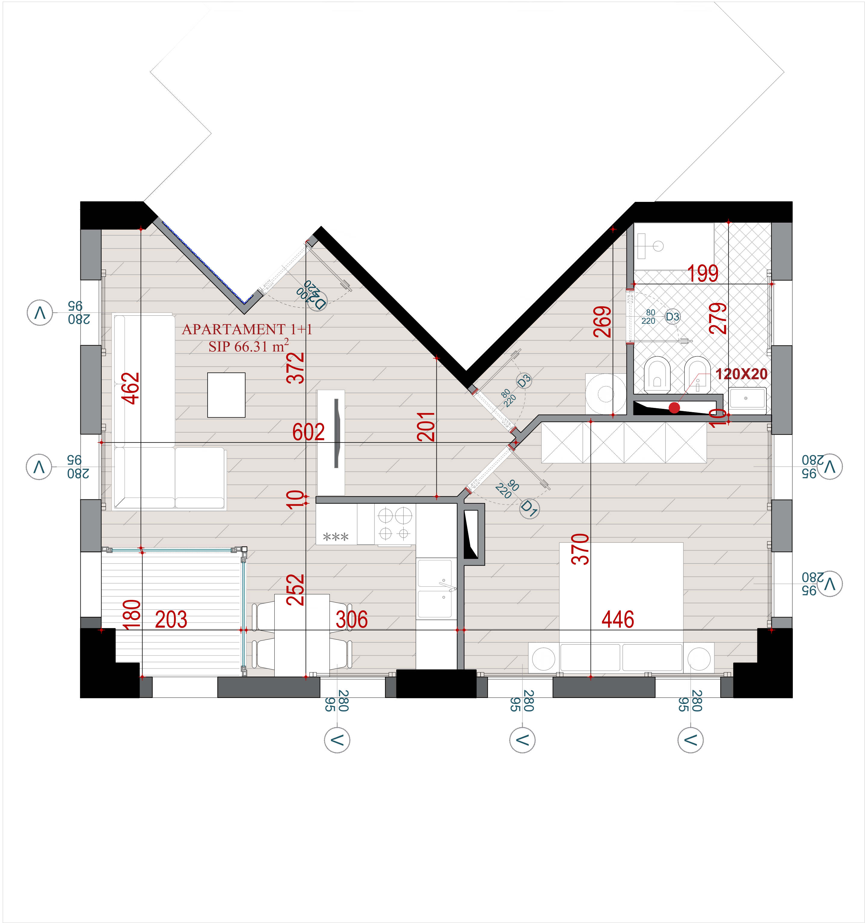
PLANIMETRIA E APARTAMENTIT NR. 23
