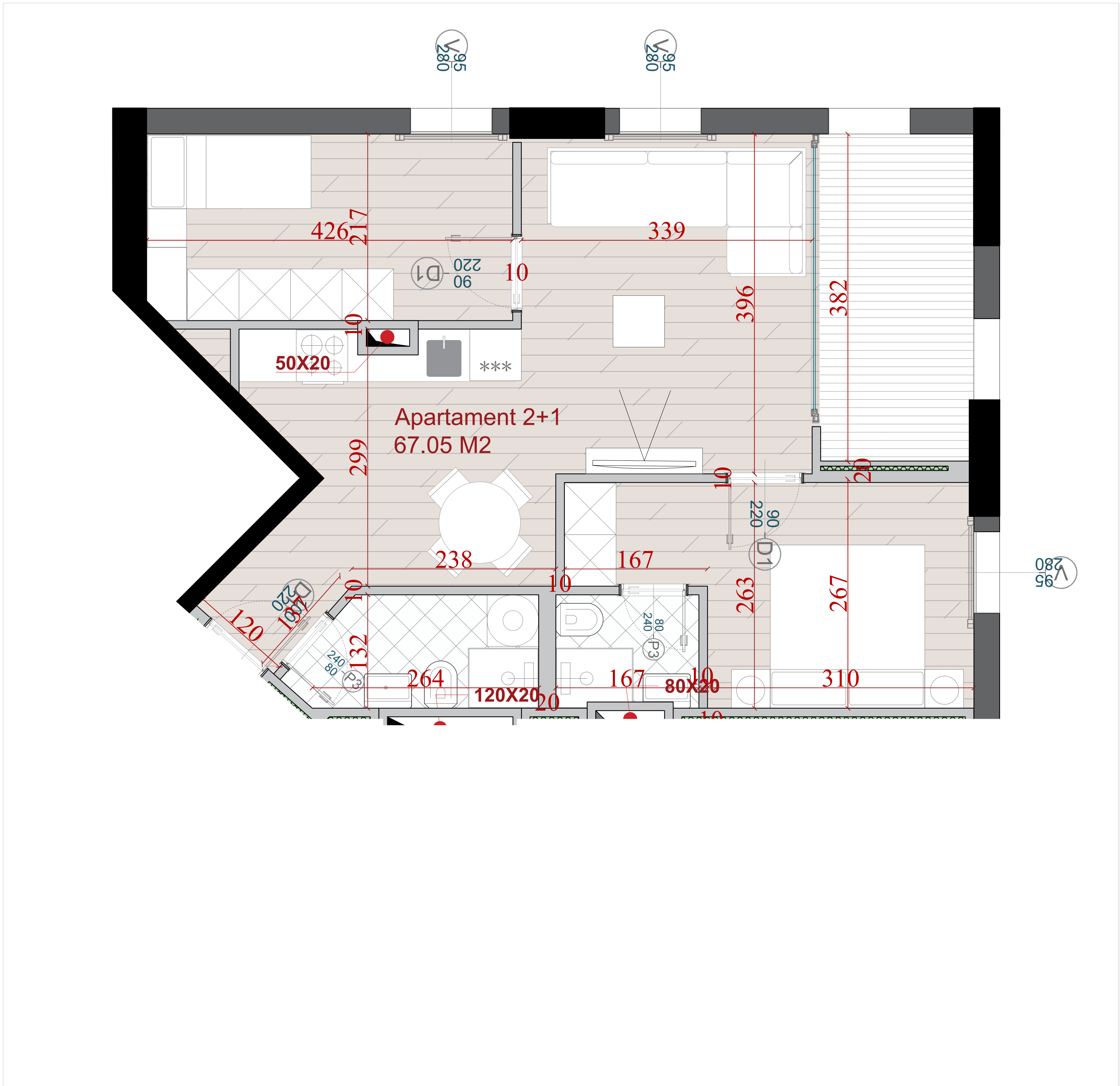
PLANIMETRIA E APARTAMENTIT NR. 39
