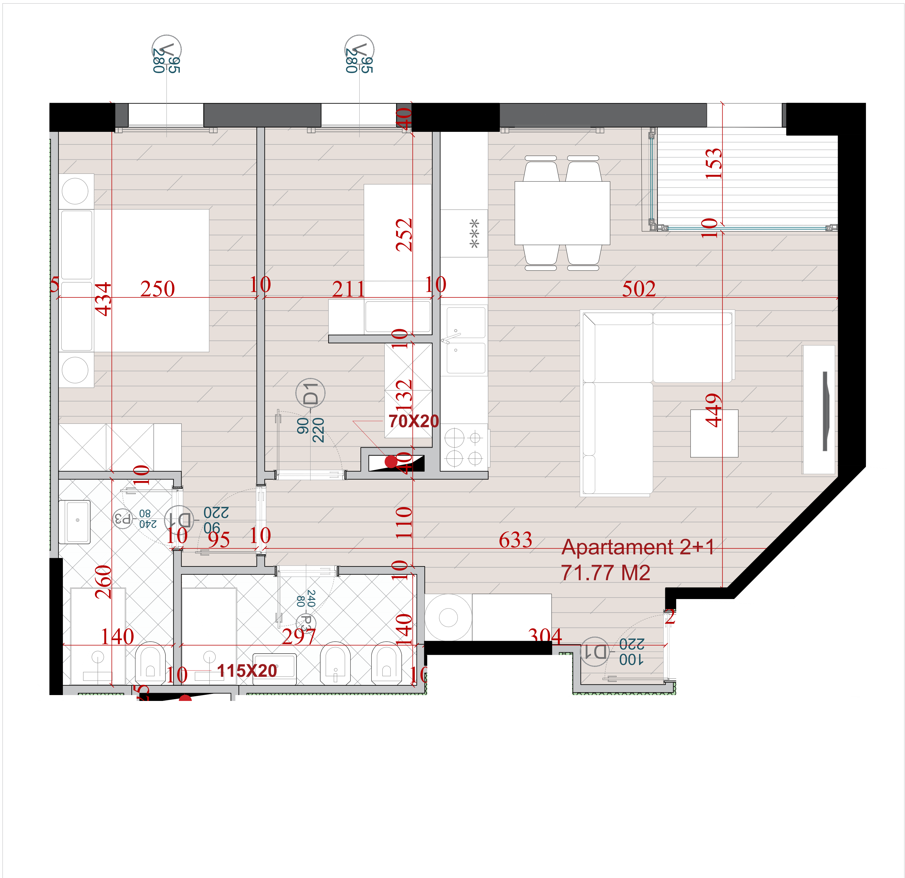
PLANIMETRIA E APARTAMENTIT NR. 38
