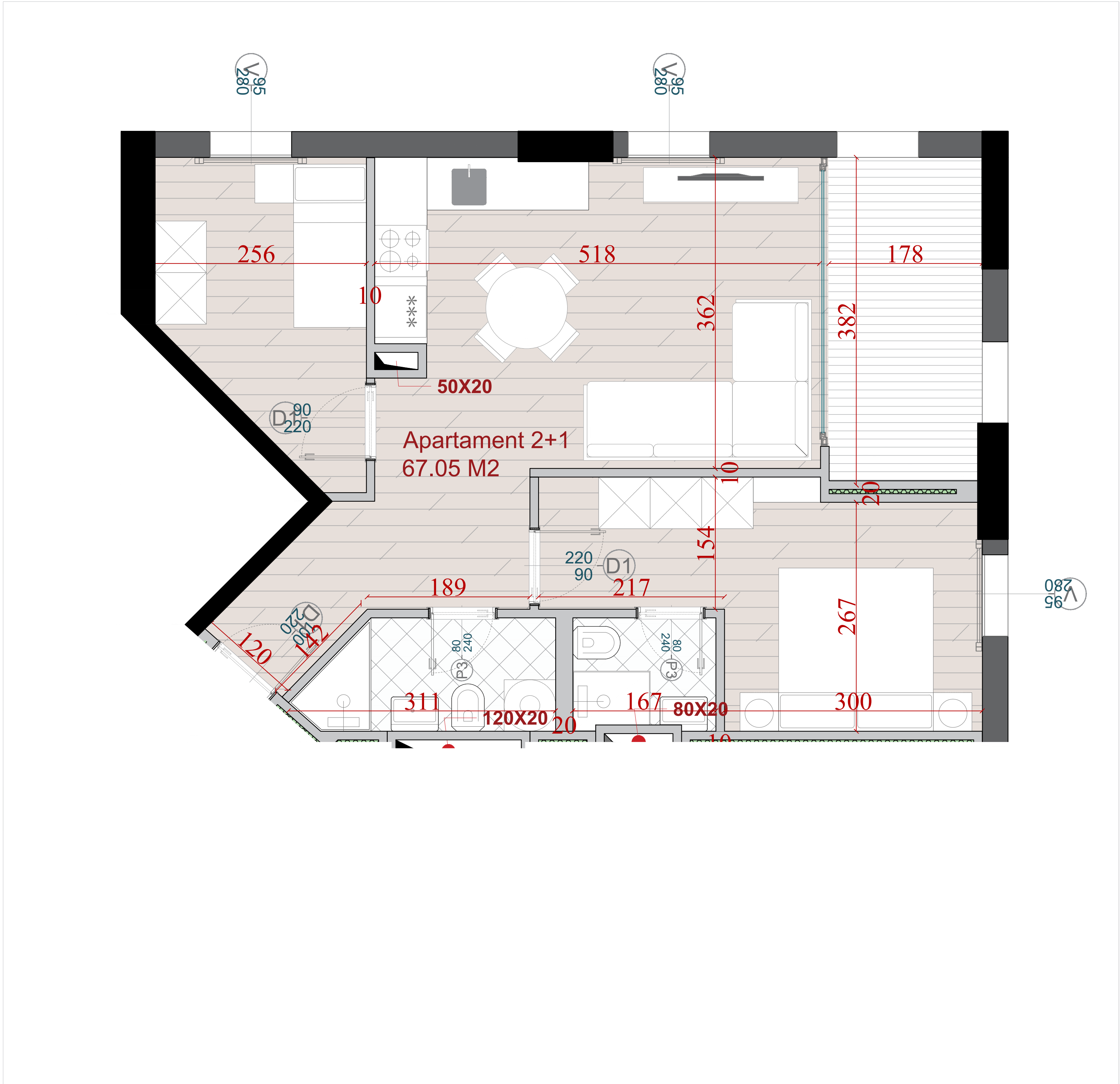
PLANIMETRIA E APARTAMENTIT NR. 35
