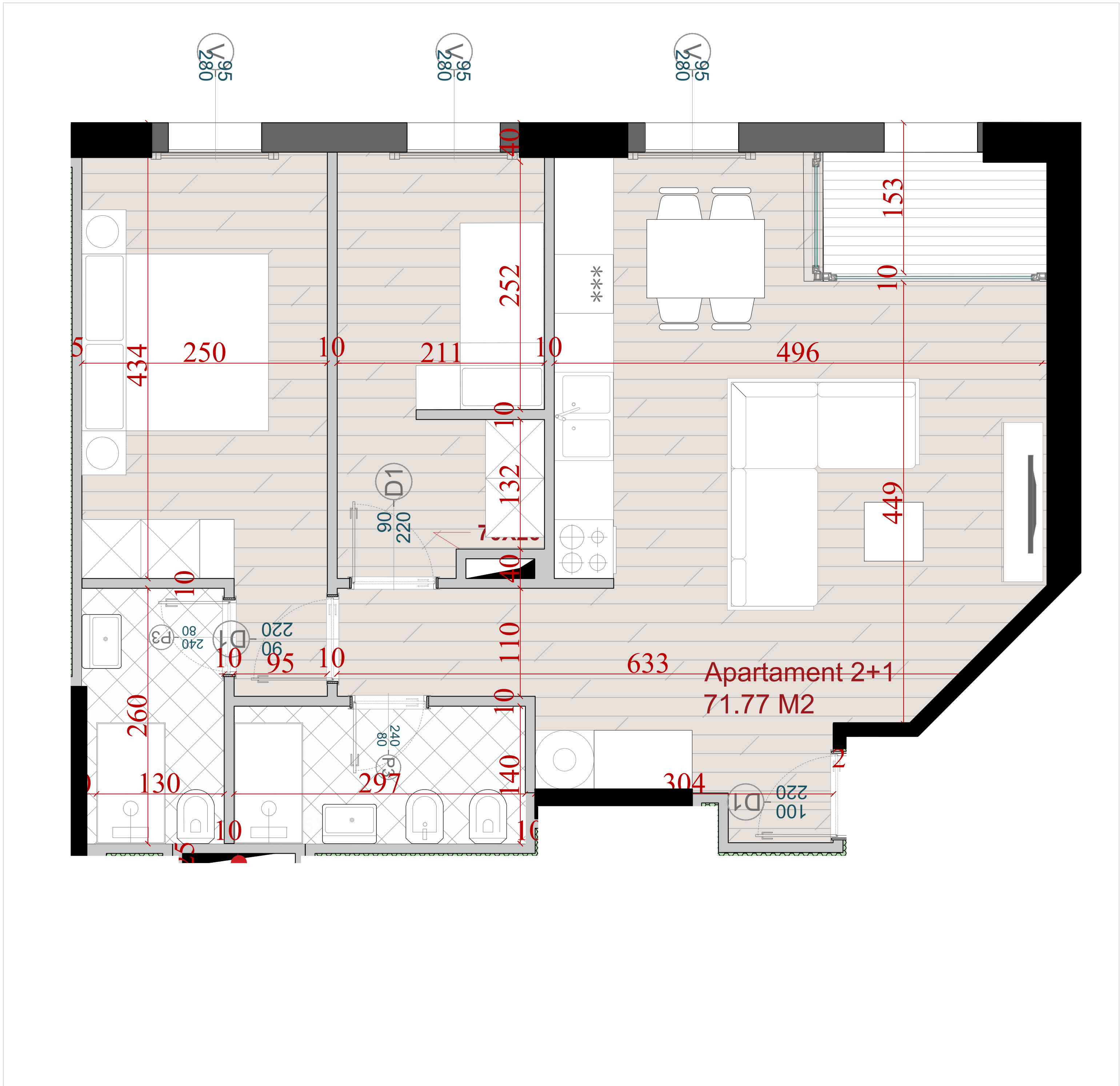
PLANIMETRIA E APARTAMENTIT NR. 34
