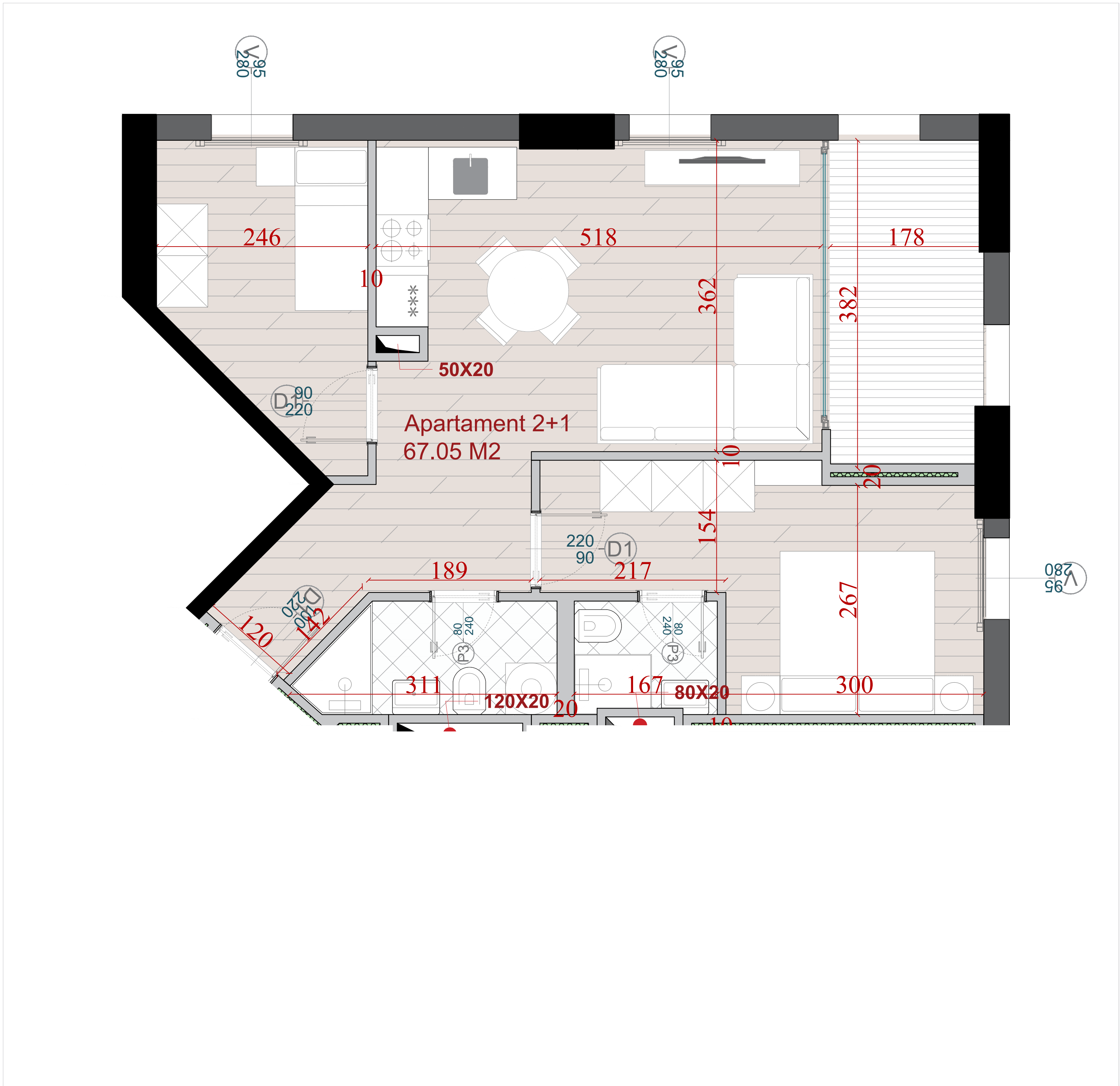
PLANIMETRIA E APARTAMENTIT NR. 31
