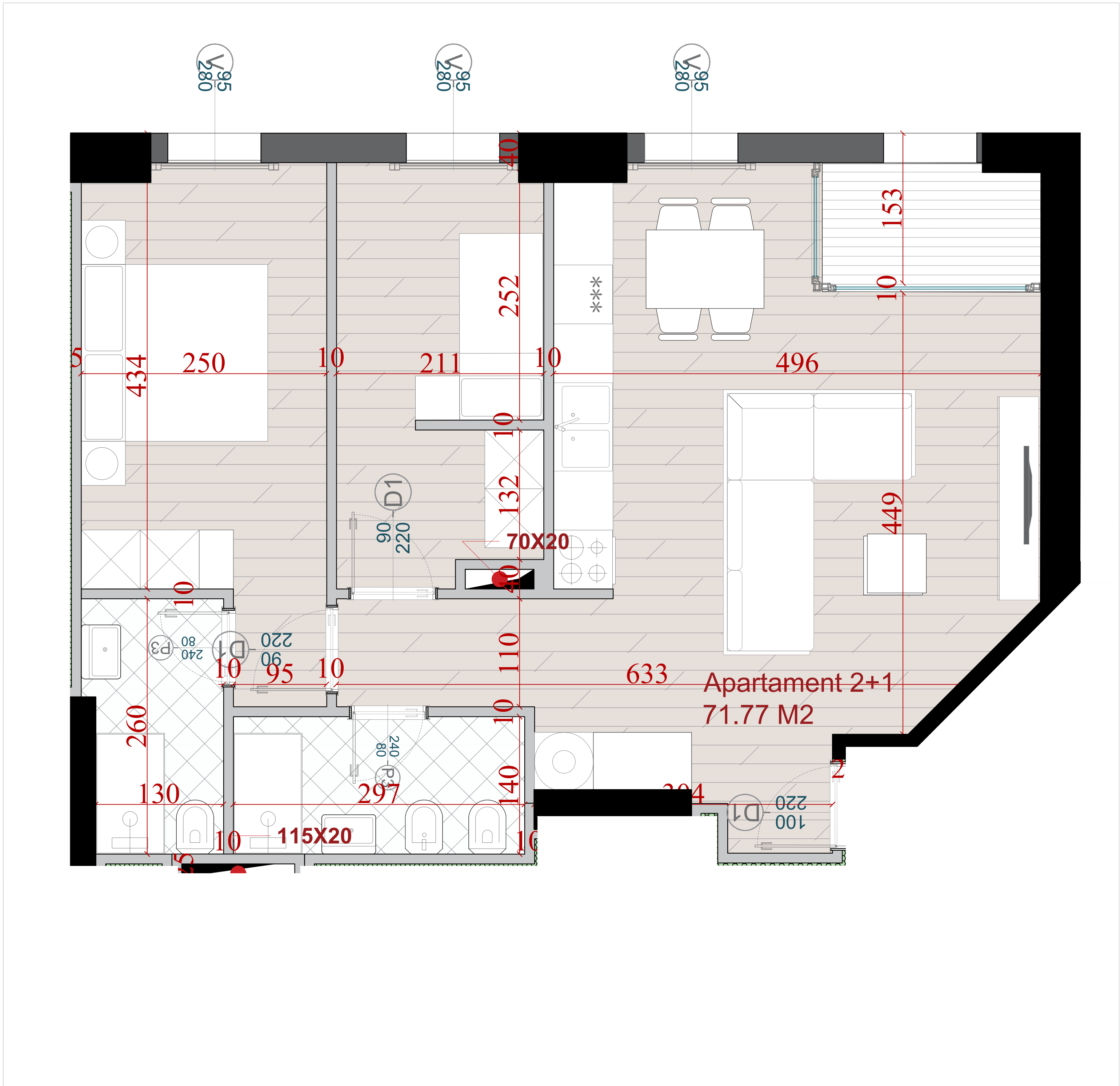
PLANIMETRIA E APARTAMENTIT NR. 14
