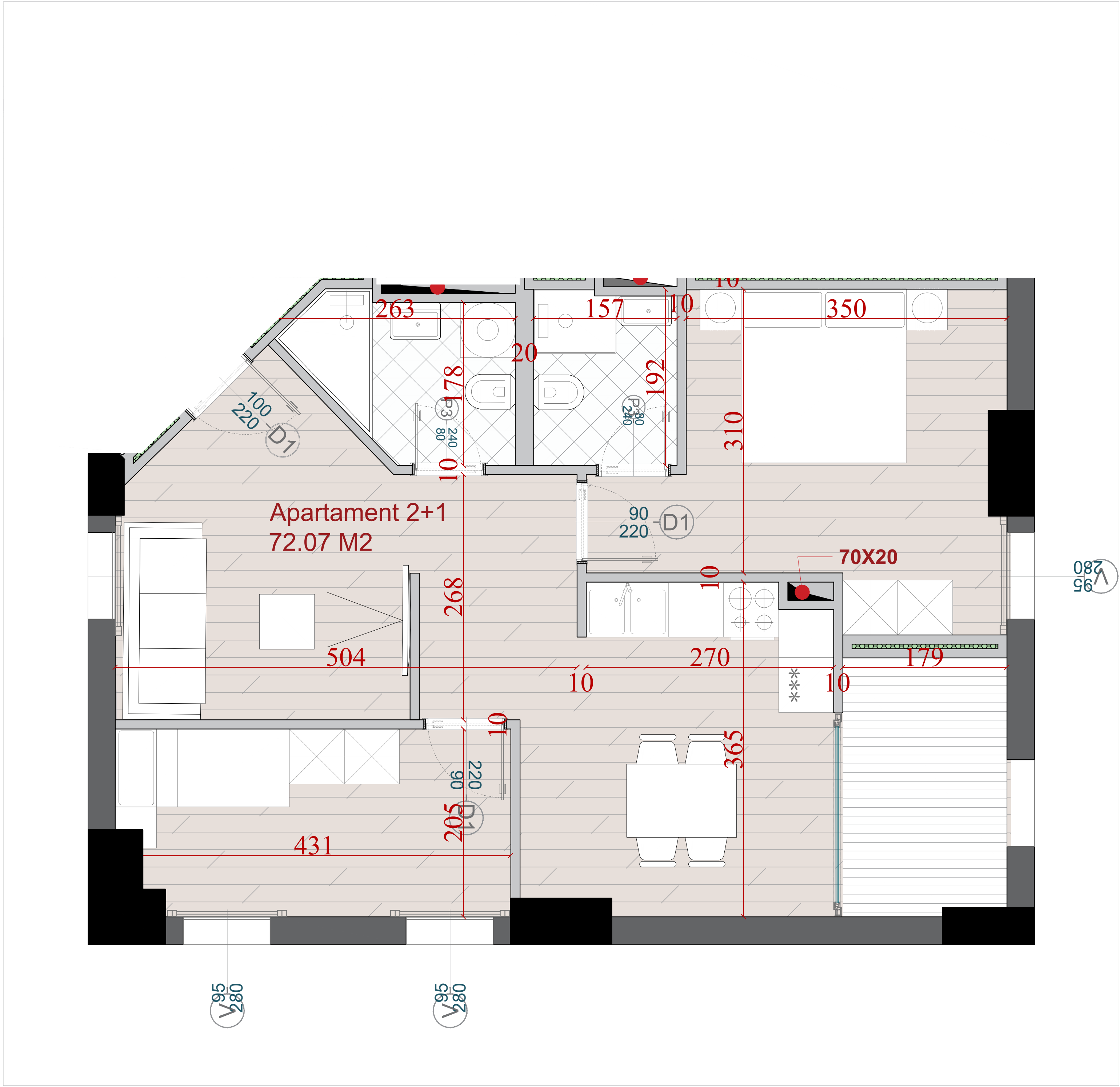
PLANIMETRIA E APARTAMENTIT NR. 12
