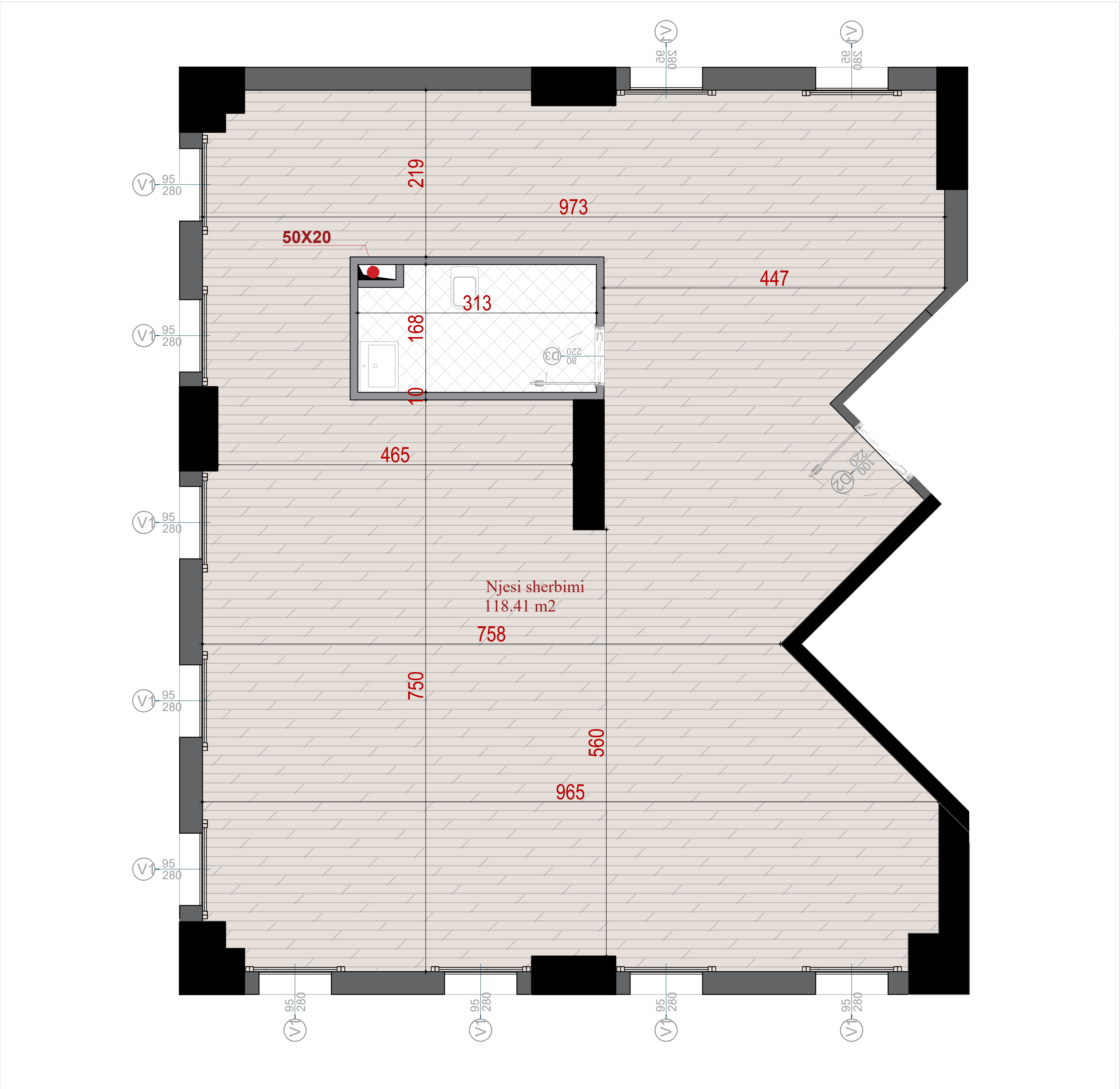
PLANIMETRIA E SHERBIMIT NR.02
