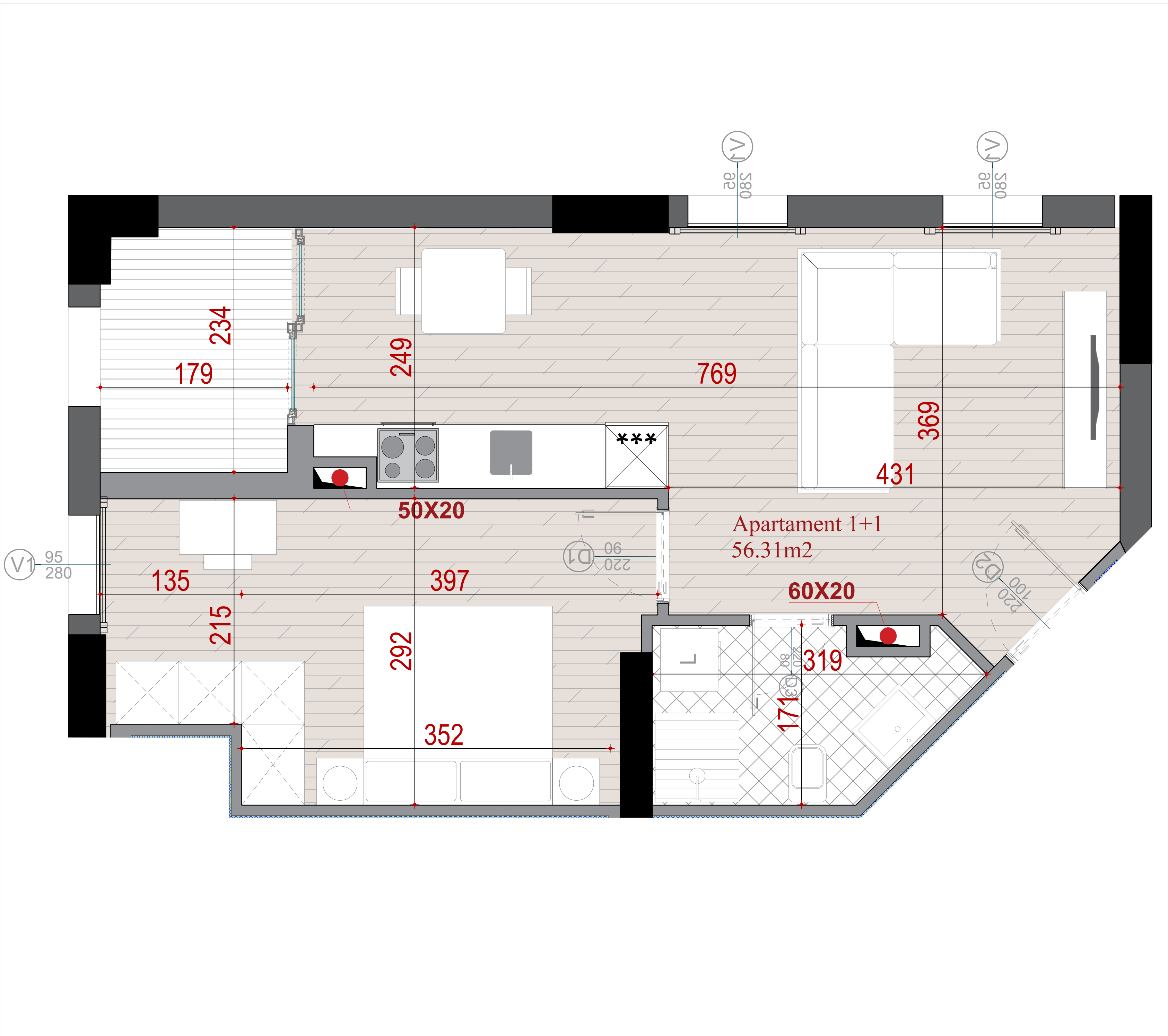
PLANIMETRIA E APARTAMENTIT NR. 19
