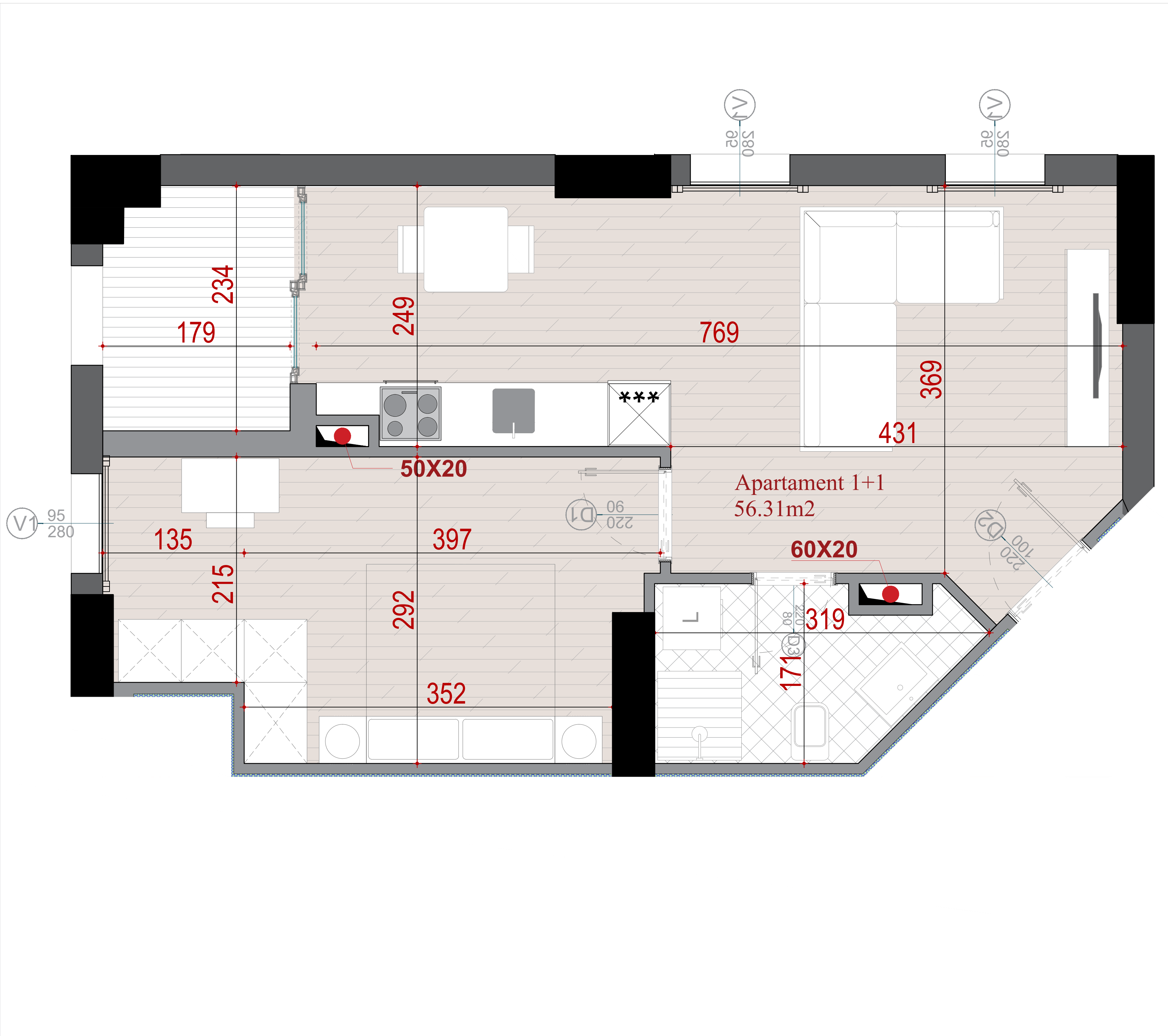
PLANIMETRIA E APARTAMENTIT NR. 13
