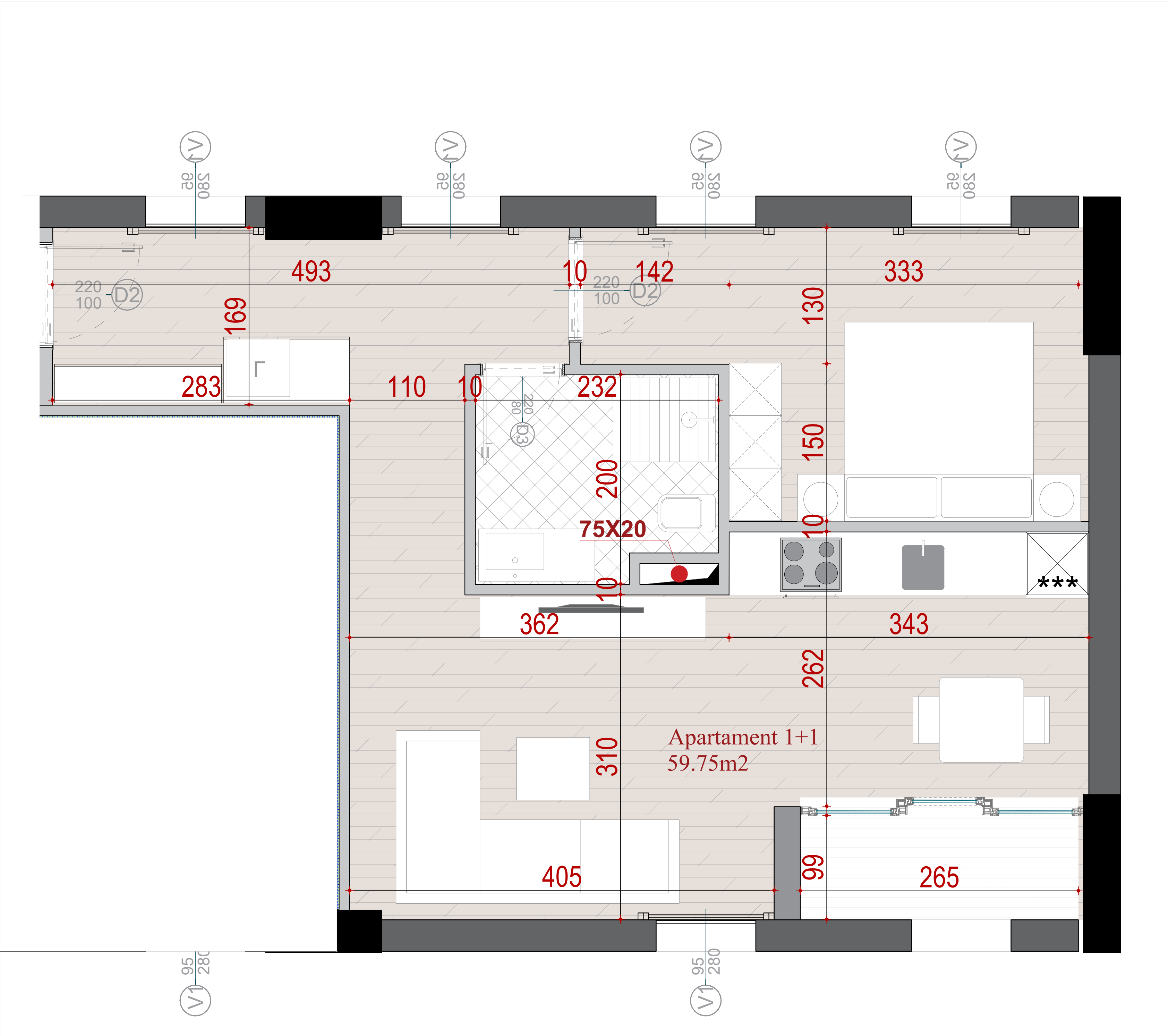
PLANIMETRIA E APARTAMENTIT NR. 12
