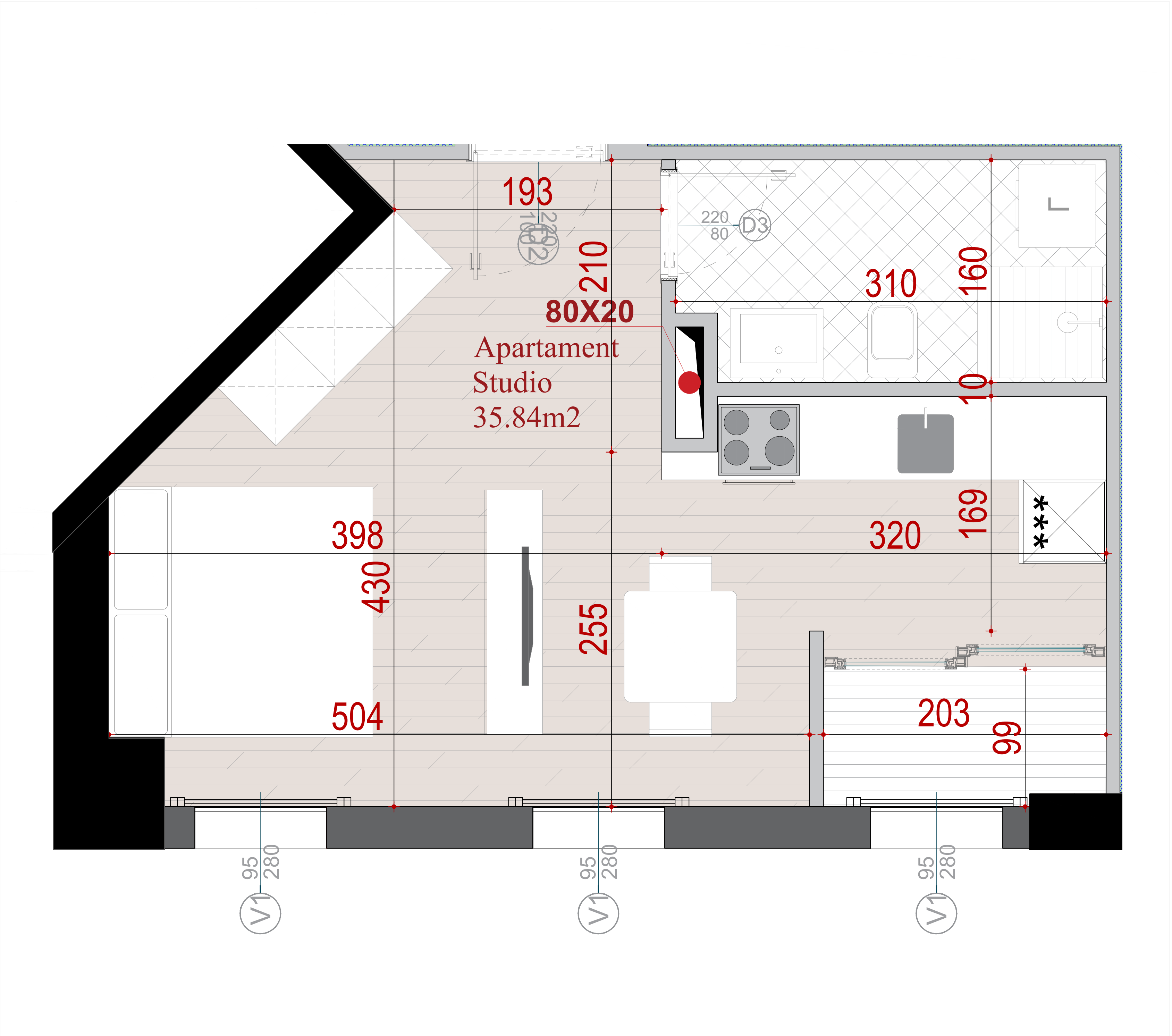
PLANIMETRIA E APARTAMENTIT NR. 11
