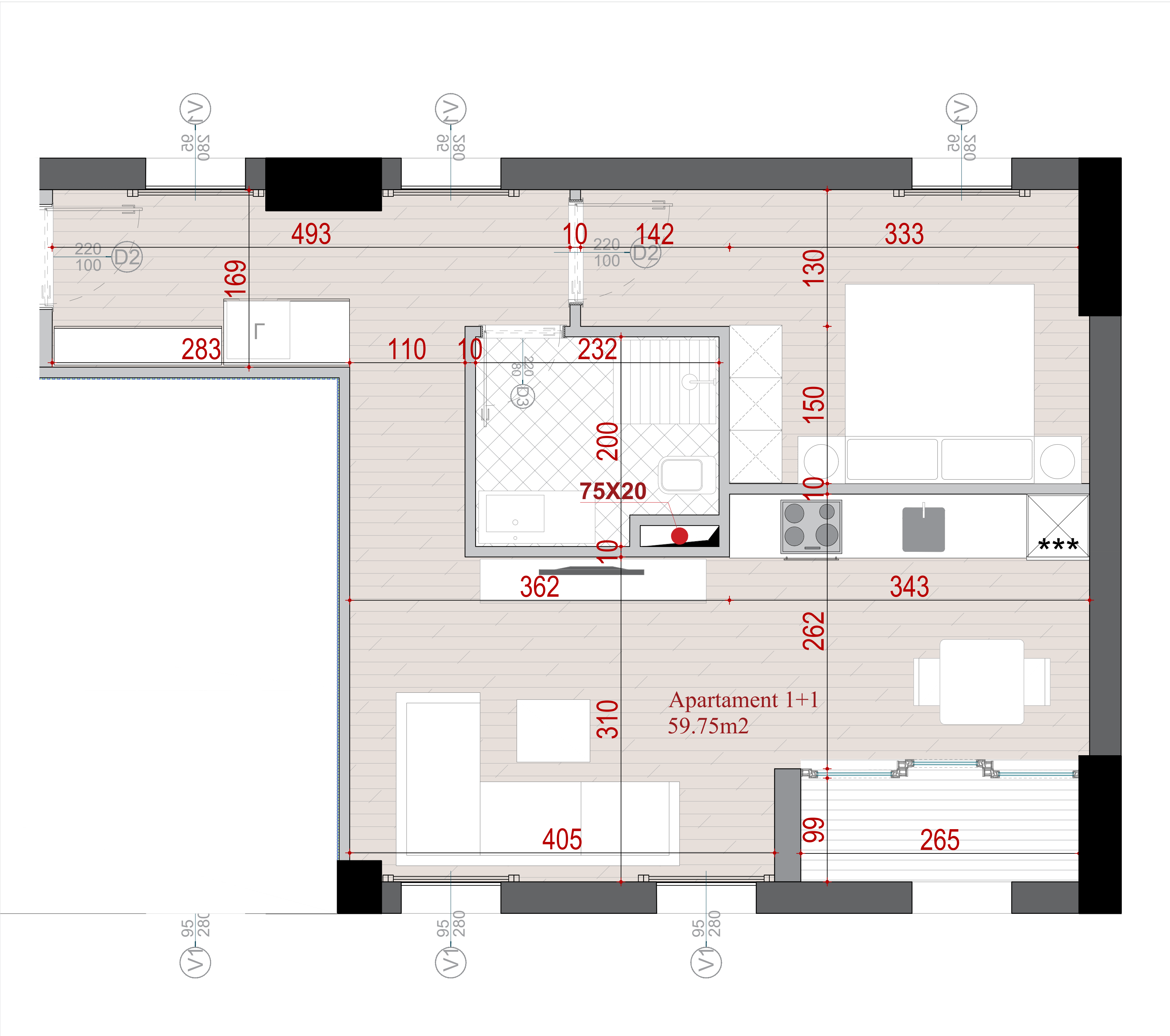
PLANIMETRIA E APARTAMENTIT NR. 08
