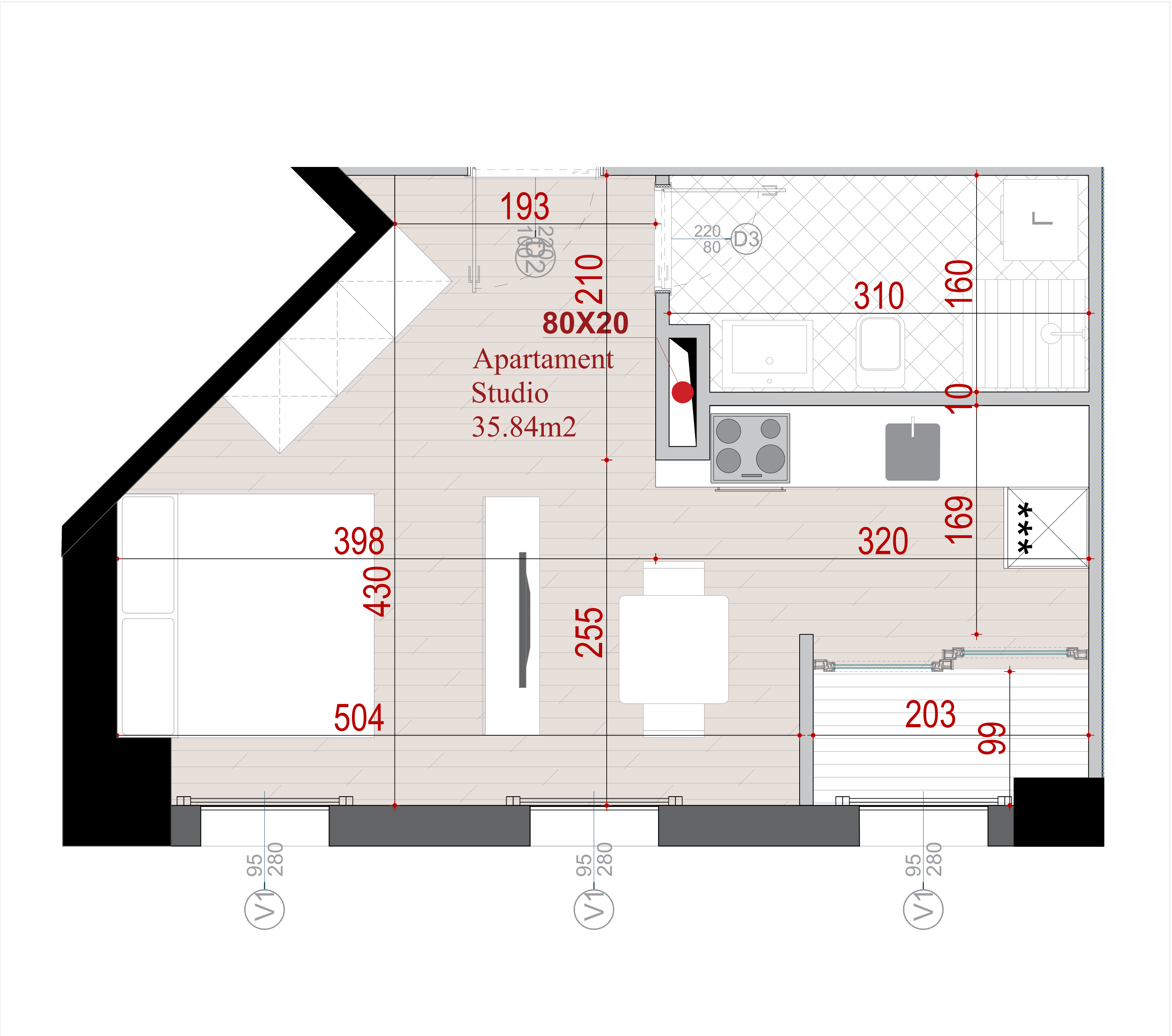
PLANIMETRIA E APARTAMENTIT NR. 03
