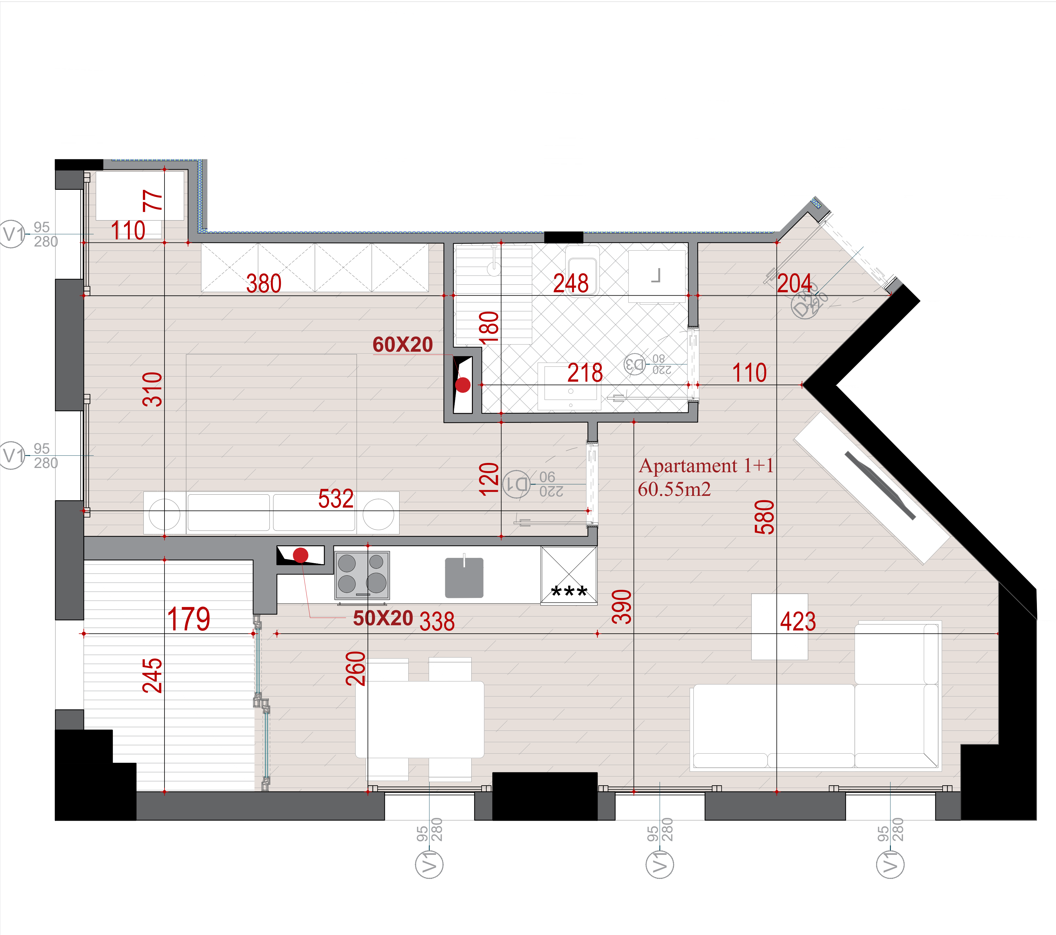
PLANIMETRIA E APARTAMENTIT NR. 02
