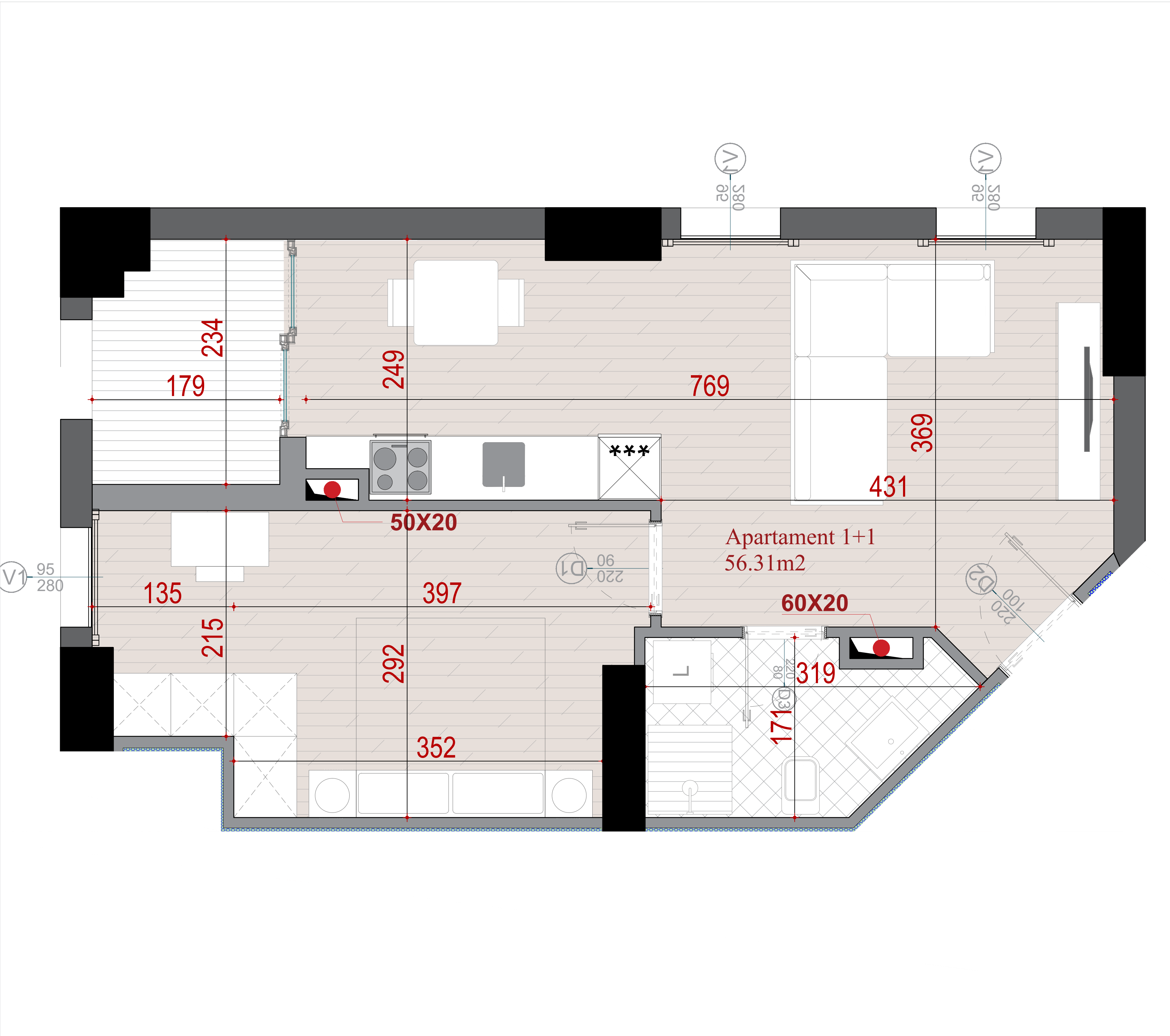
PLANIMETRIA E APARTAMENTIT NR. 01
