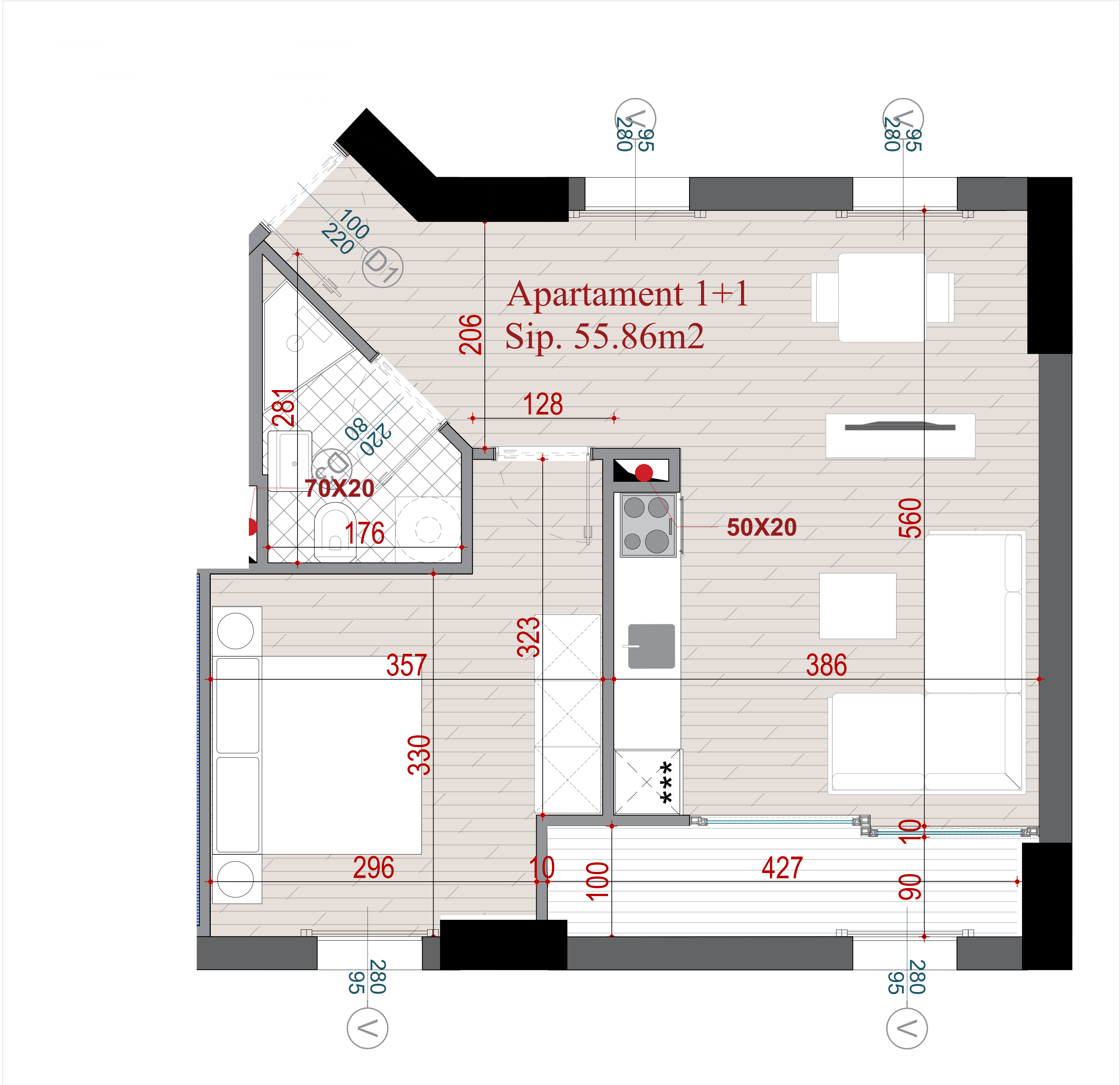
PLANIMETRIA E APARTAMENTIT NR. 25
