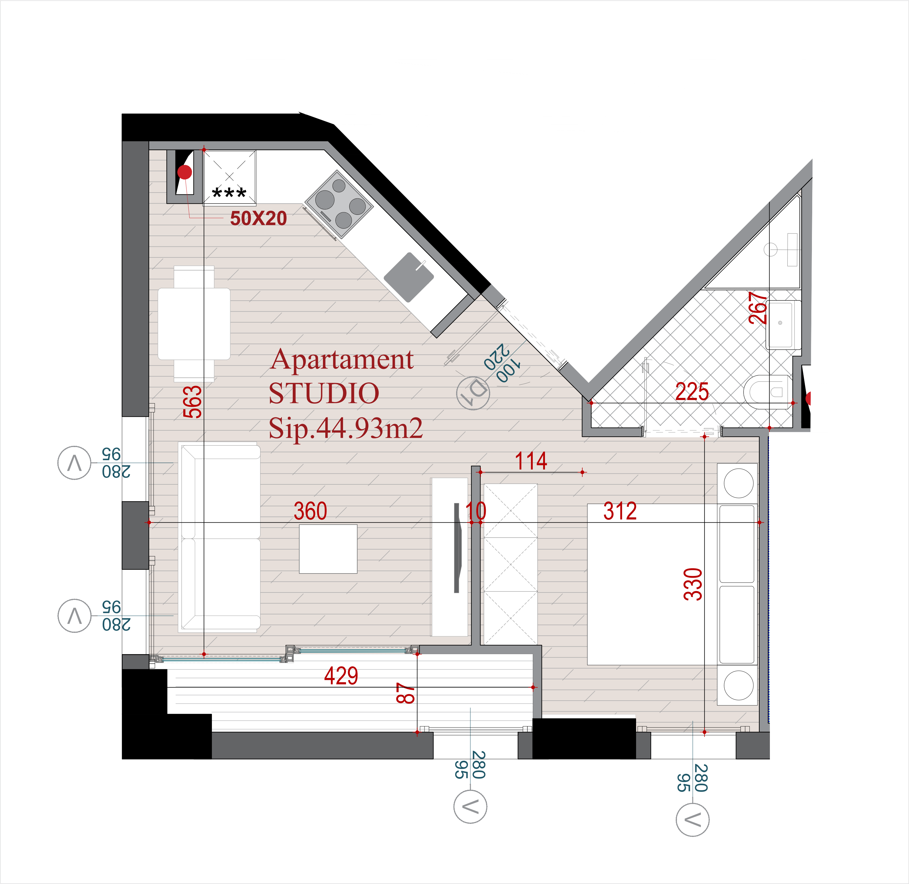
PLANIMETRIA E APARTAMENTIT NR. 22
