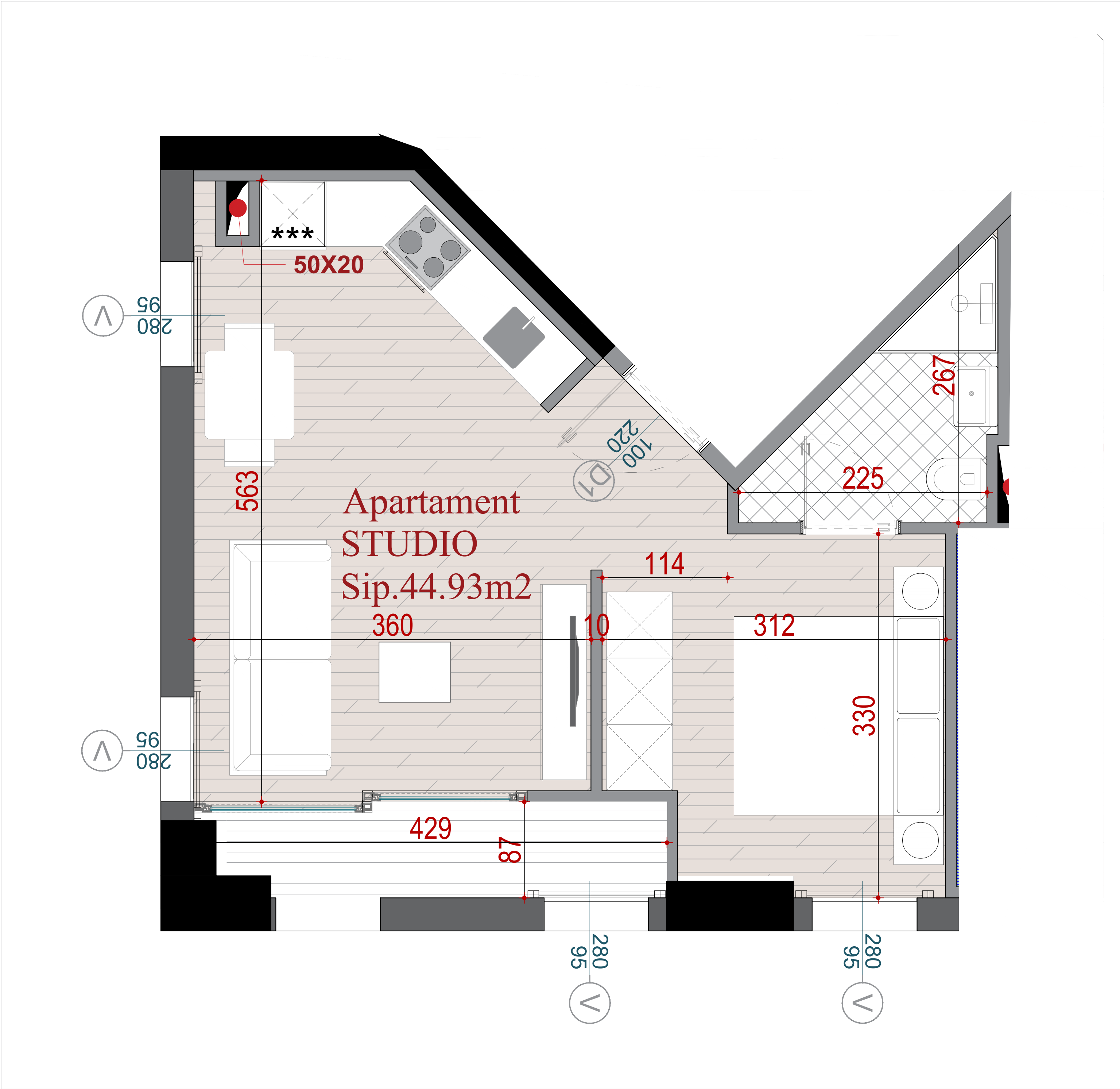
PLANIMETRIA E APARTAMENTIT NR. 18
