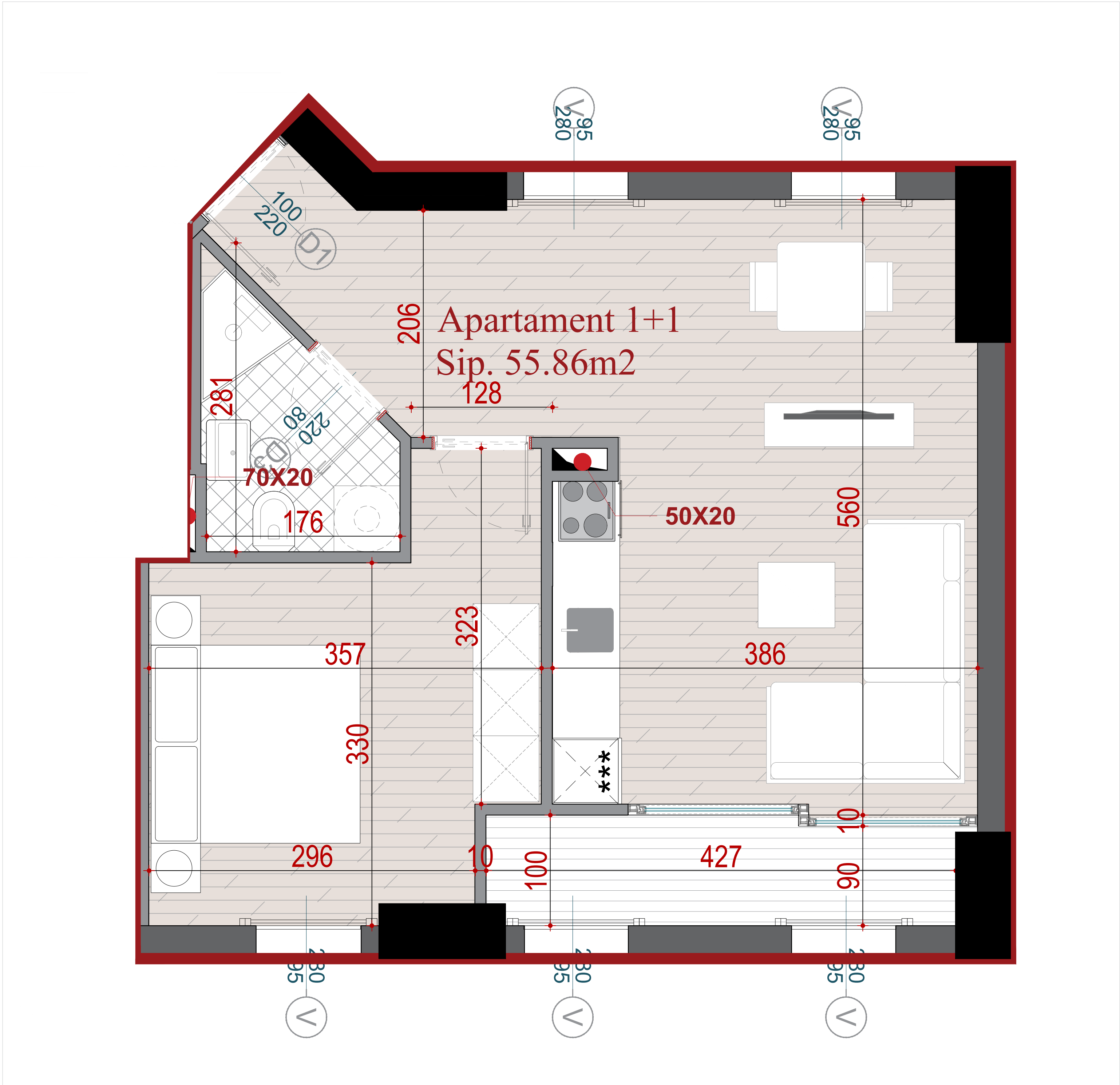
PLANIMETRIA E APARTAMENTIT NR. 13
