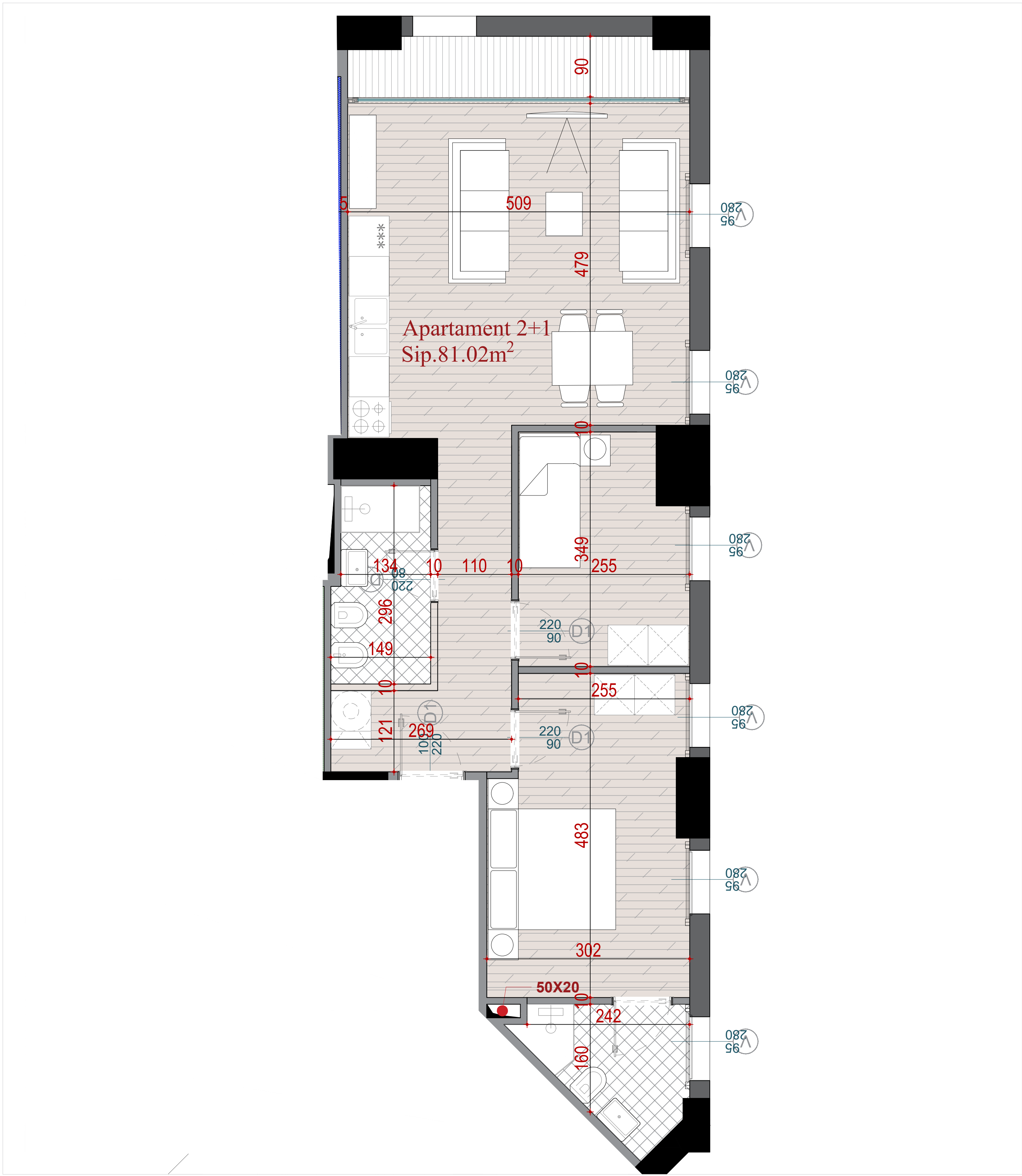
PLANIMETRIA E APARTAMENTIT NR. 04
